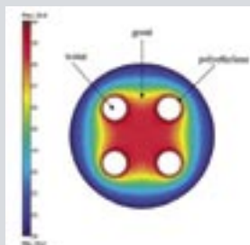
SONDA - numerični model izračuna učinkovitosti geosonde
